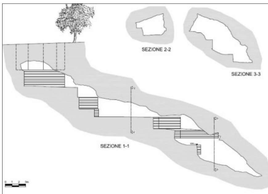
Fig. 3b - Rilievo in sezione della grotta eseguito con il laserscanner.
