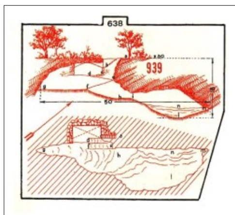
Fig. 2a - Rilievo originale tratto dal "2000 Grotte".
