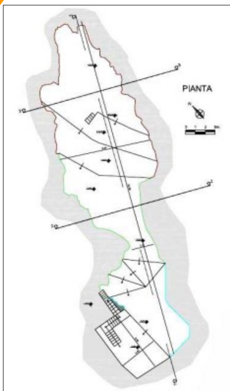
Fig. 3a - Rilievo in pianta della grotta eseguito con il laserscanner.
