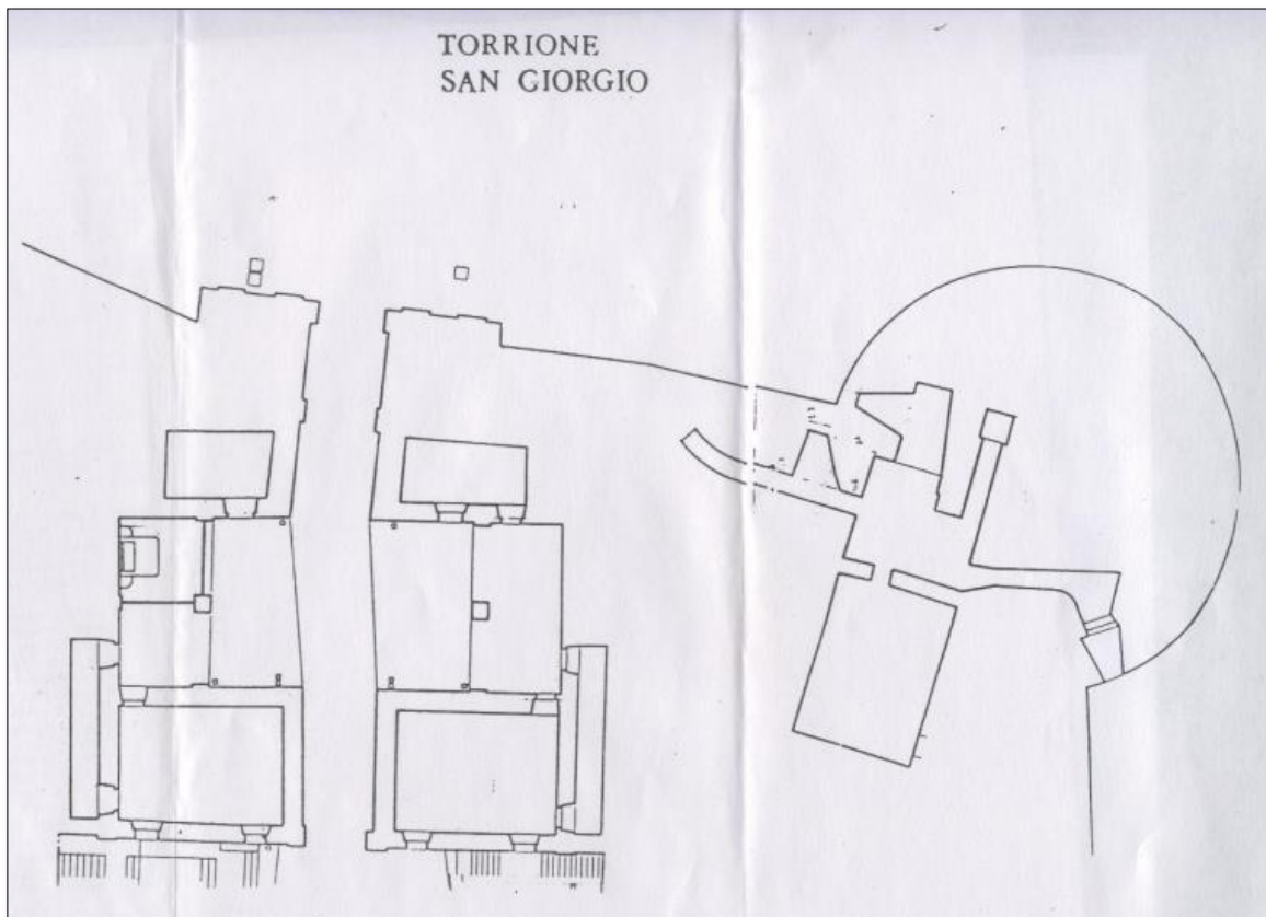
Fig. 82 - Pianta del Torrione San Giorgio con riferimento alla Porta Nuova. Si può notare il cunicolo, all'interno del torrione, che prosegue parallelamente alla cinta muraria in direzione della porta. Probabilmente le mura di Gradisca erano tutte percorse da un camminamento interno che ne collegava i torrioni.
