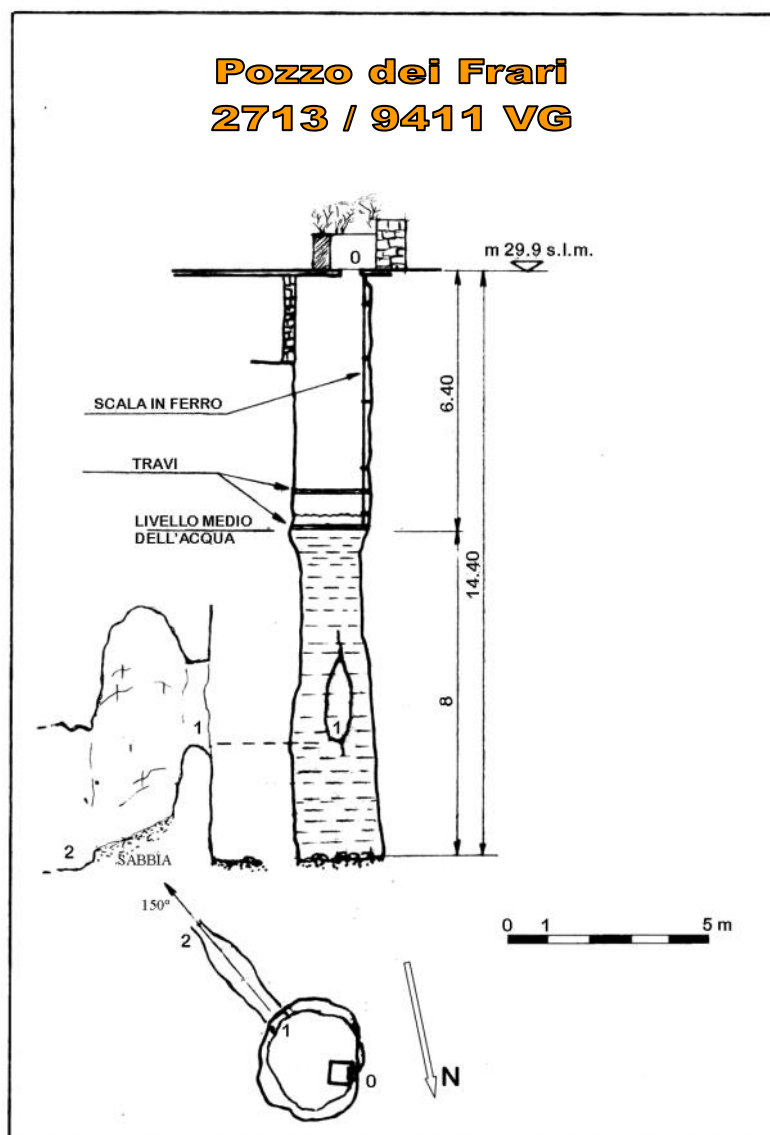
Fig. 34 - L'ultimo rilievo aggiornato del Pozzo dei Frari eseguito il 06.10.2020.
