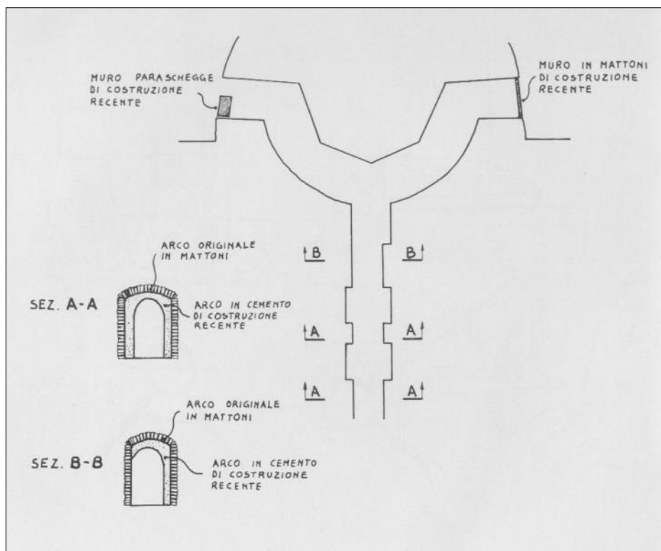
Fig. 90 - Rilievo della galleria all'interno del Torrione della Calcina (rilievo Centro Ricerche Carsiche "C. Seppenhof").
