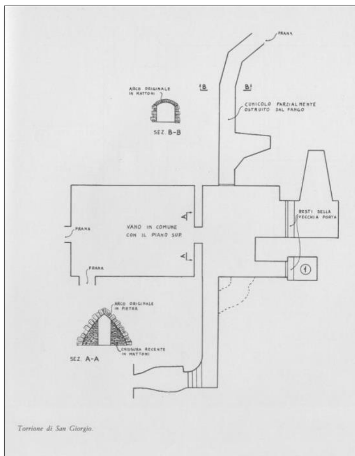
Fig. 74 - Pianta e sezioni delle parti interne al piano terra del Torrione San Giorgio (rilievo C.R.C. “C. Seppenhof”).
