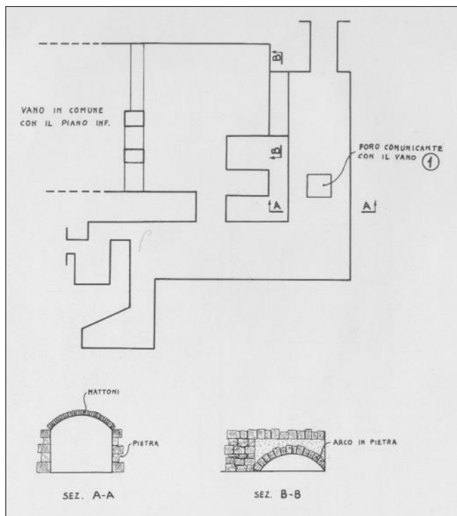
Fig. 76 - Pianta, a livello +3.98, dettaglio dei vani interni al Torrione San Giorgio il punto I (cerchiato) si riferisce alla fig. 74 (rilievo C.R.C. "C. Seppenhof").
