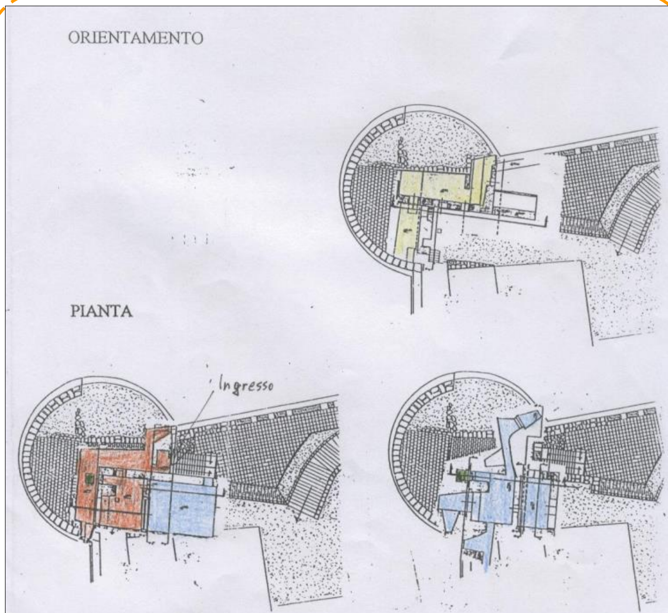
Fig. 79 - Pianta del Torrione San Giorgio in cui si possono vedere le situazioni dei vani interni su più livelli. In giallo a livello + 6.75; in marrone a livello + 3.98; in azzurro a livello + 0.
