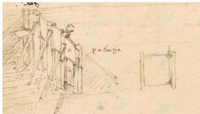
Fig. 65 - "Serraglio mobile": diga di ritenuta e paratoie mobili da aprire in caso di invasioni turche (Manoscritti B, f. 64 recto)
